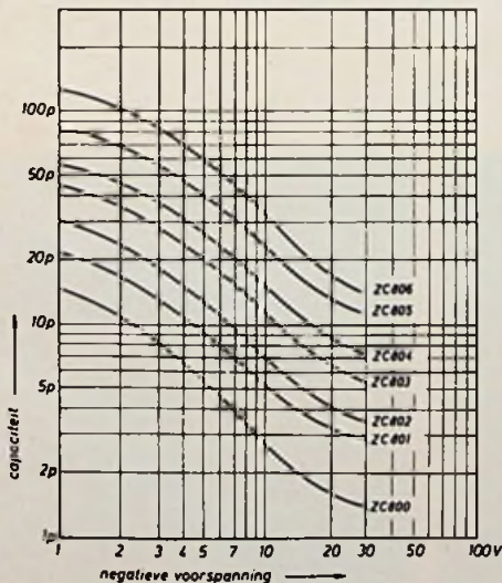
Fig. 9. Capaciteit/spanningverhouding van de ZC800 serie hyper abrupte afstemdioden.
